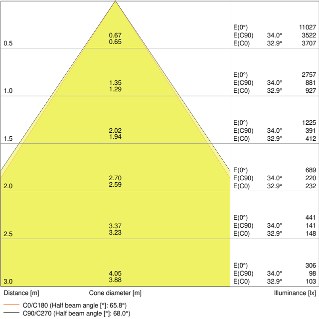
LN INDV D 1200 34W 3000K TH
